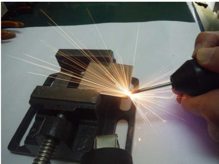
肉盛り加工
